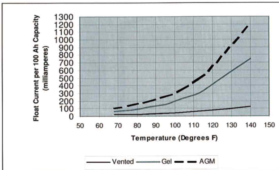
< Fig. 1. 온도에 따른 충전 전류 변화 >
